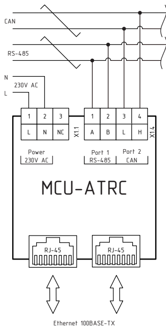
Схема подключения MCU-ATRC
