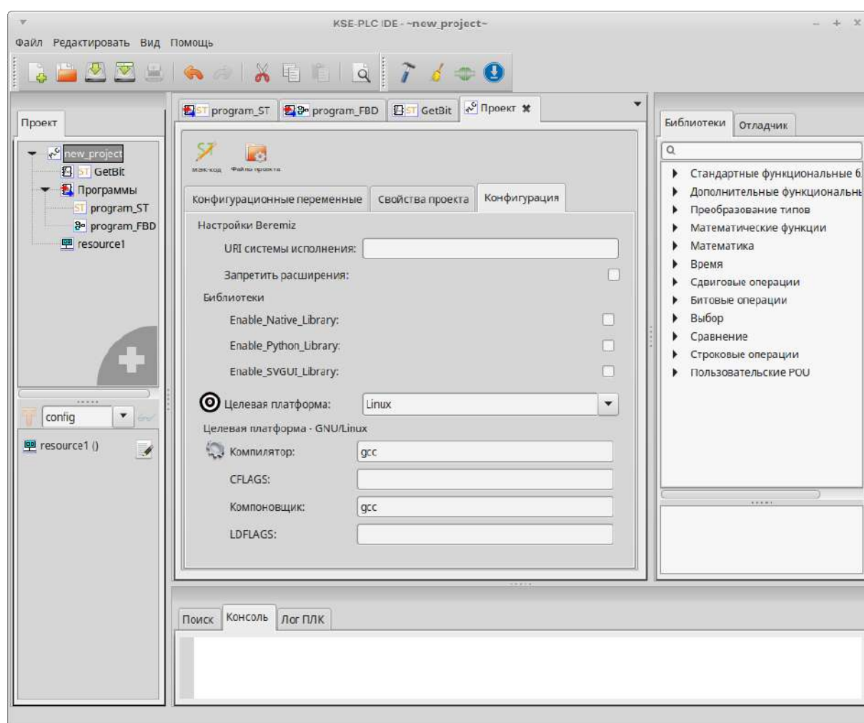
Рисунок 1 - Настройка проекта
