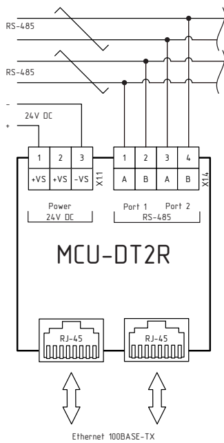
Схема подключения MCU-DT2R
